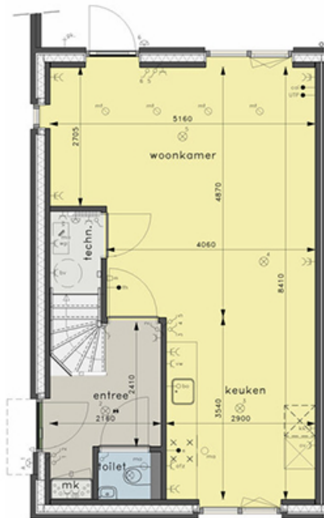
BEGANE GROND
