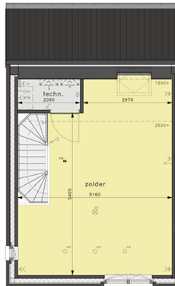
2E VERDIEPING
