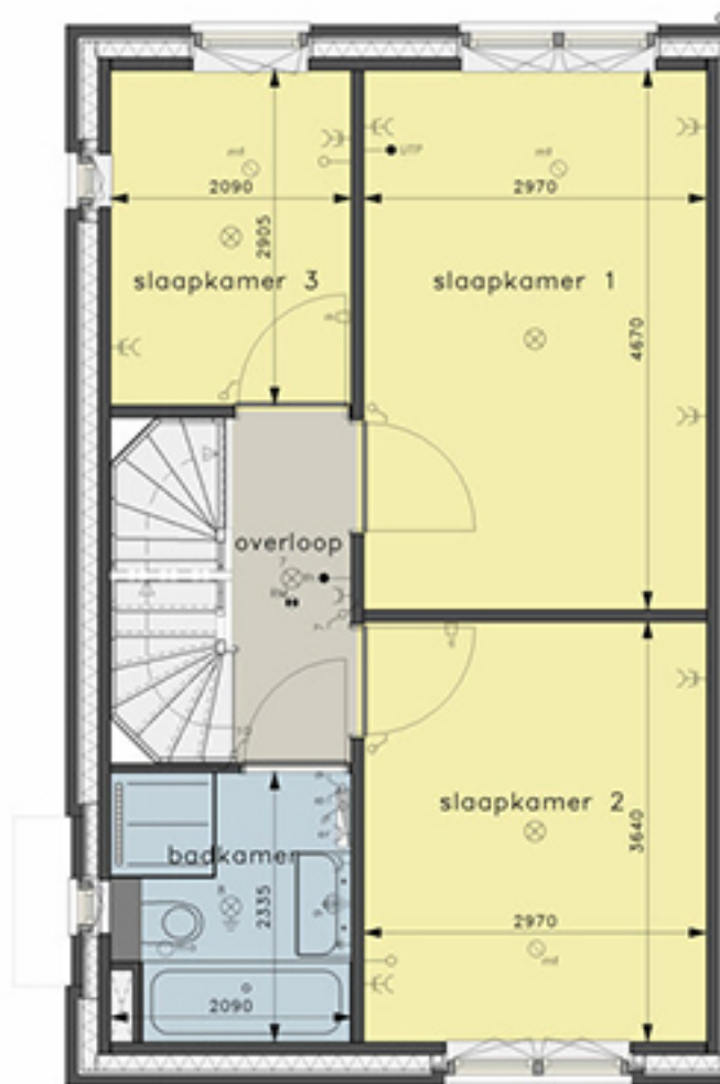
1E VERDIEPING
