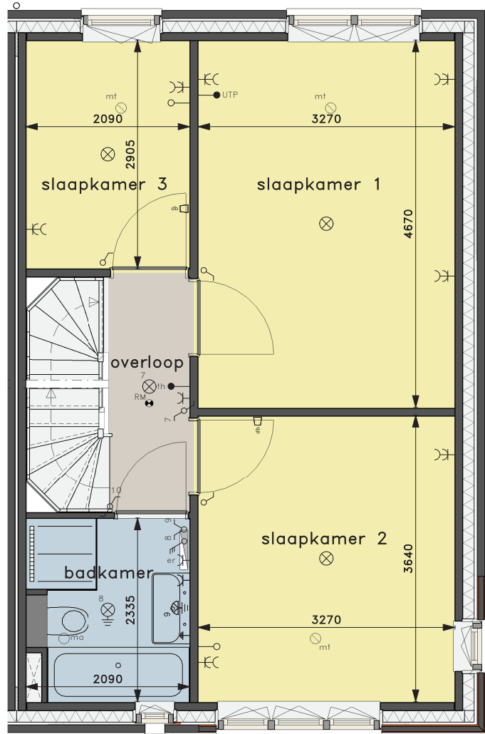
1E VERDIEPING
