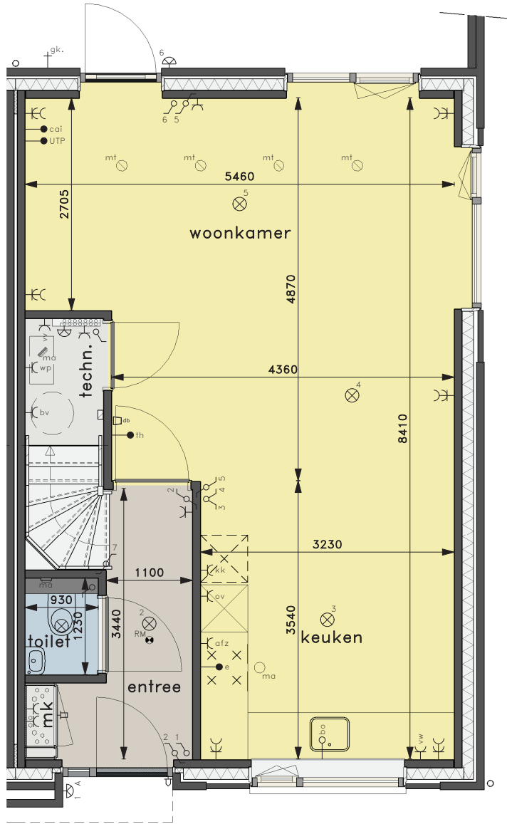
BEGANE GROND
